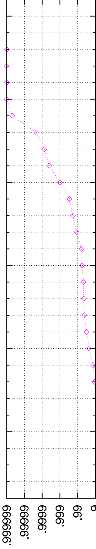
pos-files-cdf.ep
