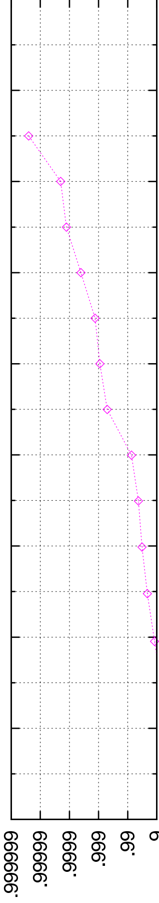
dirents-dirs-cdf.ep
