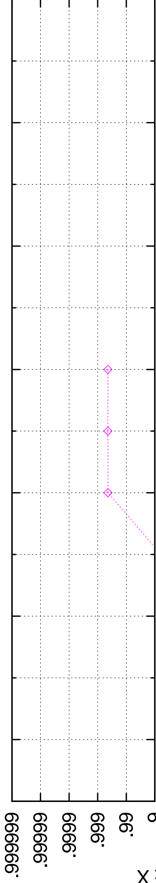
atime-bytes-cdf.ep
