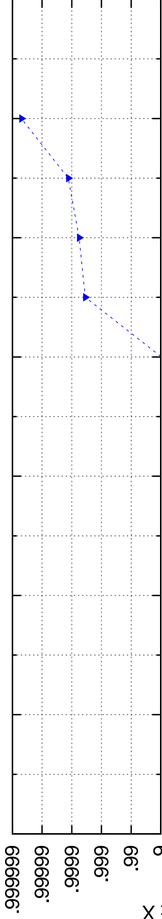
mtime-bytes-cdf.ep
