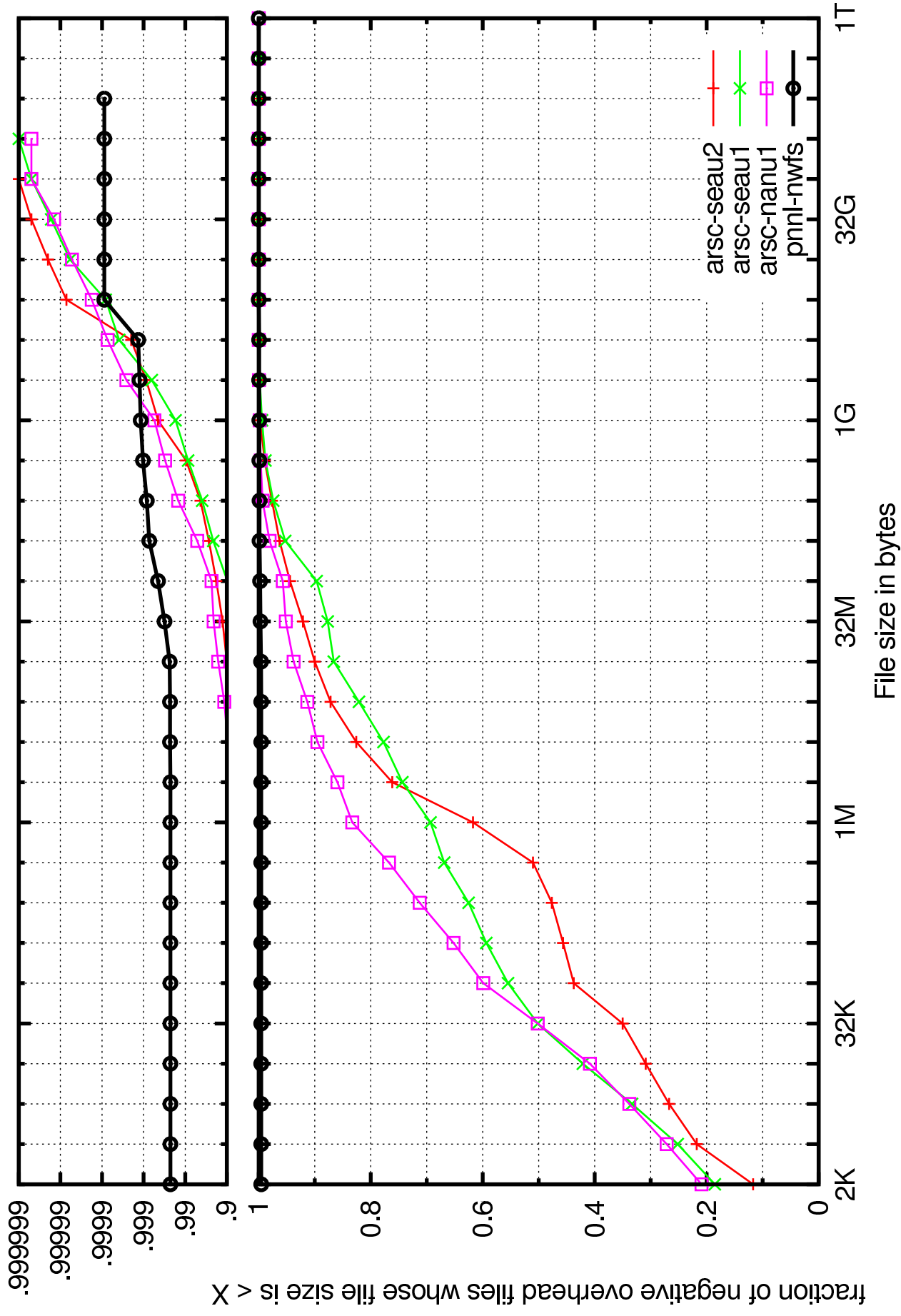
neg-files-cdf.ep
