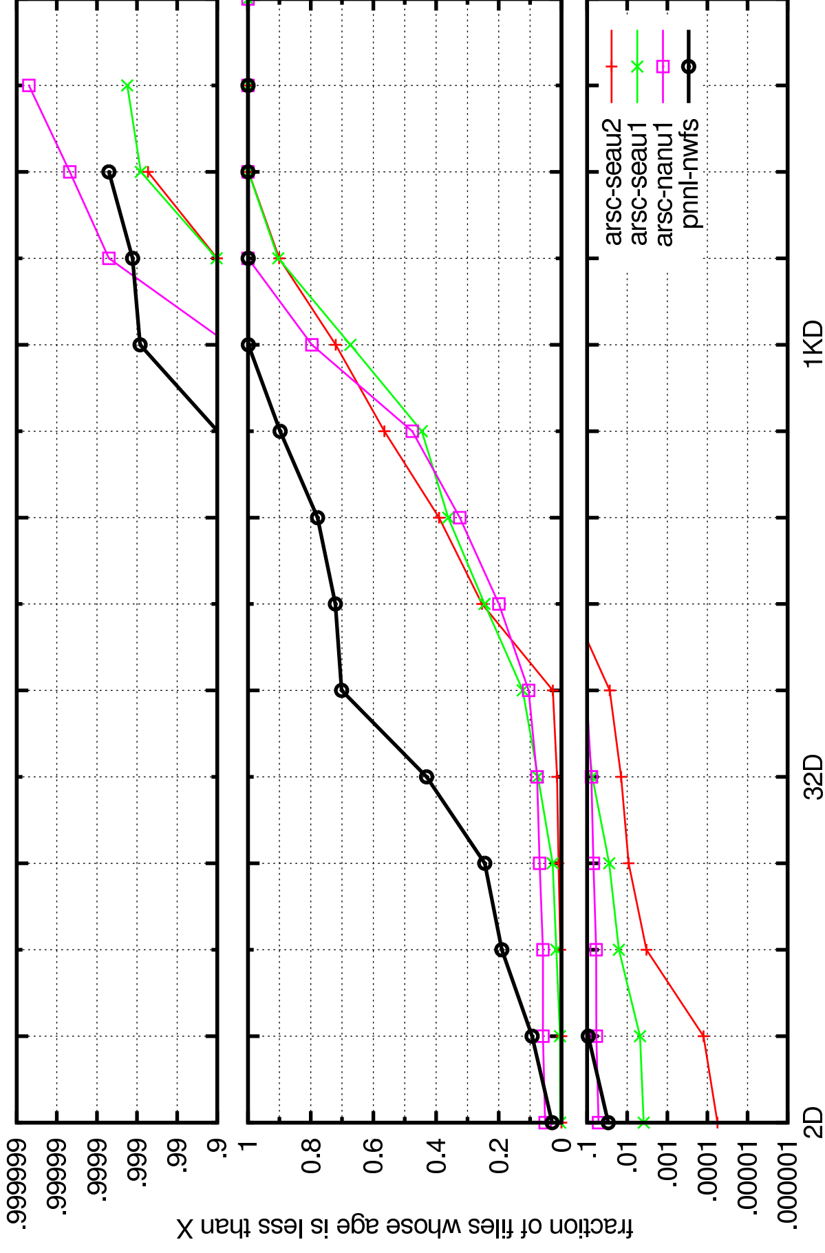
atime-files-cdf.ep
